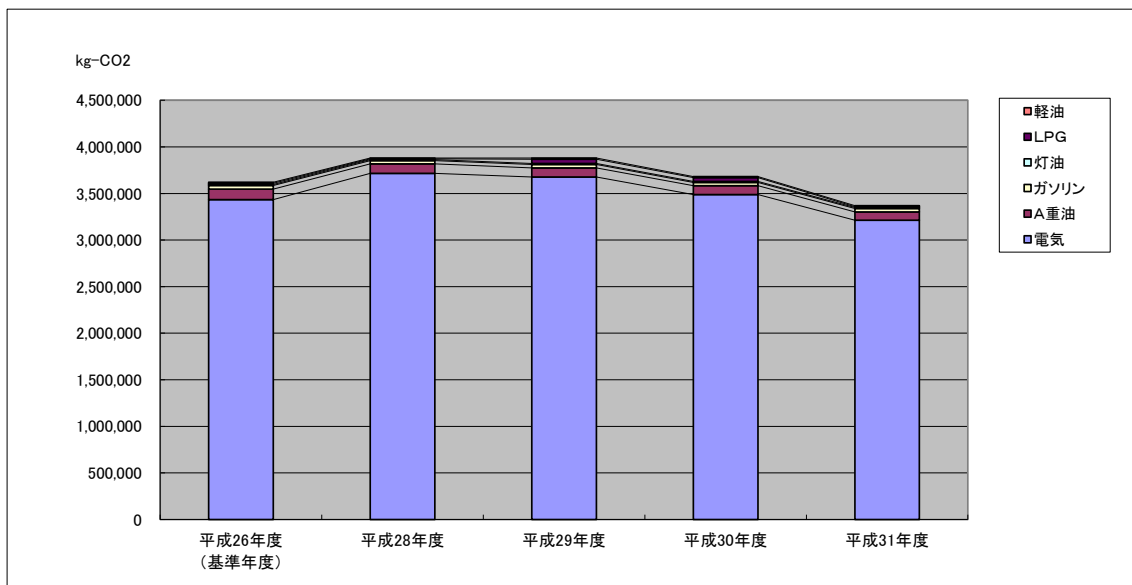
図5-3 二酸化炭素排出量
