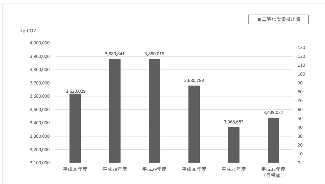
図5-1 温室効果ガス及び経年変化
